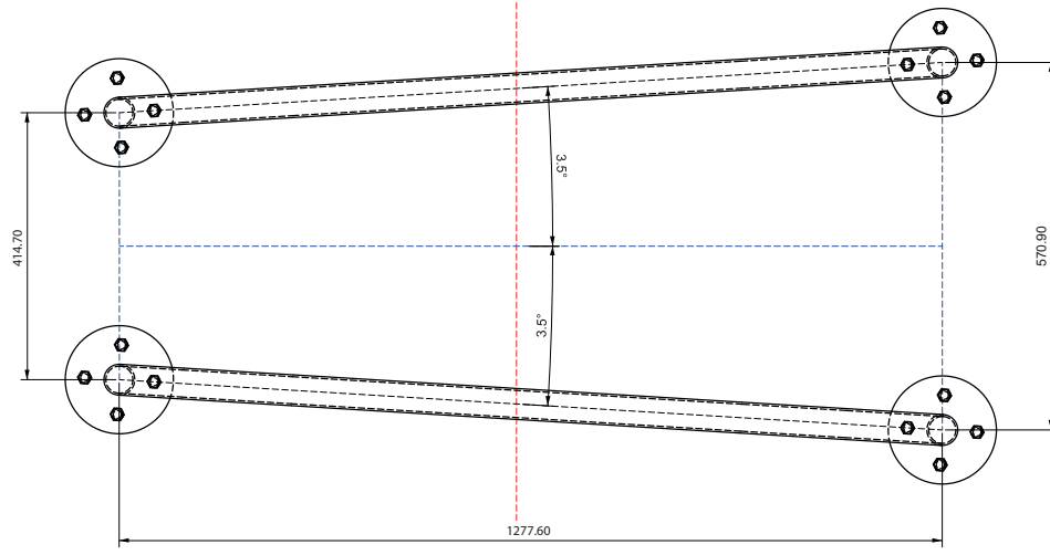
PIANTA
